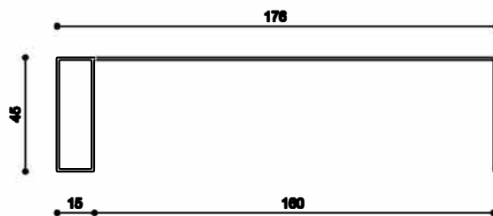
44. PIEZA VERTICAL CHAPA ENCUENTRO FACHADA
