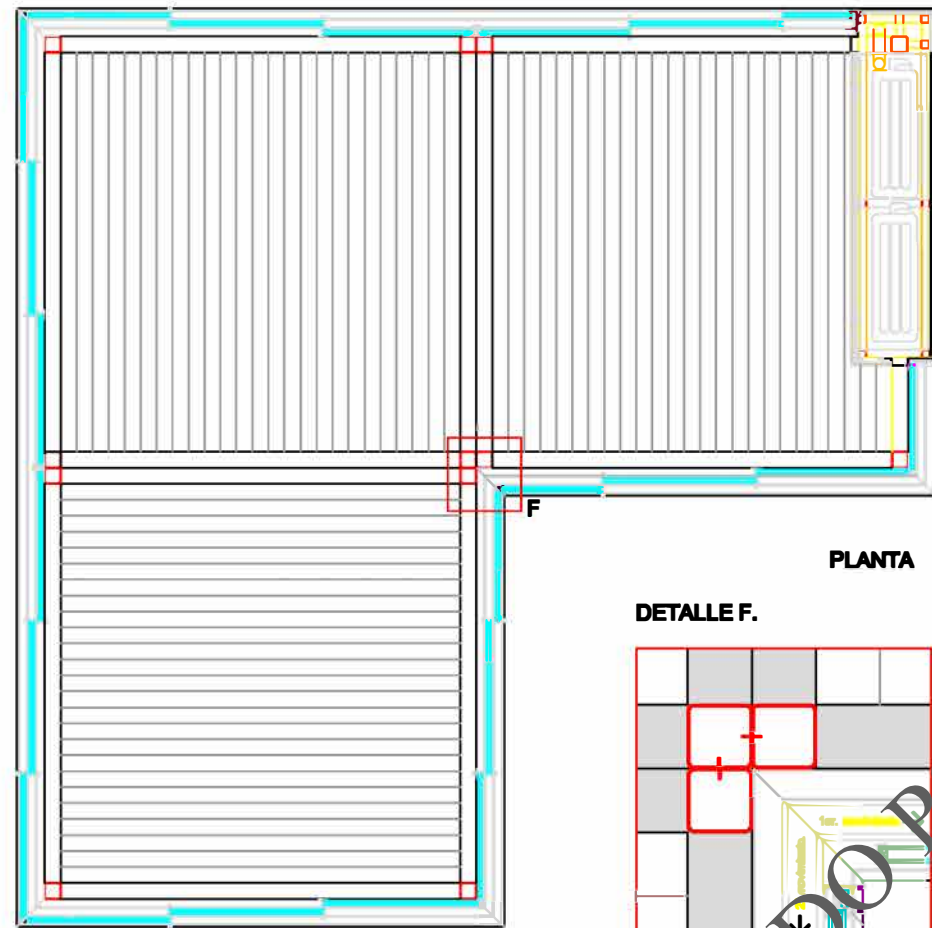
APERTURA DE CARPINTERÍA EN ESQUINA
