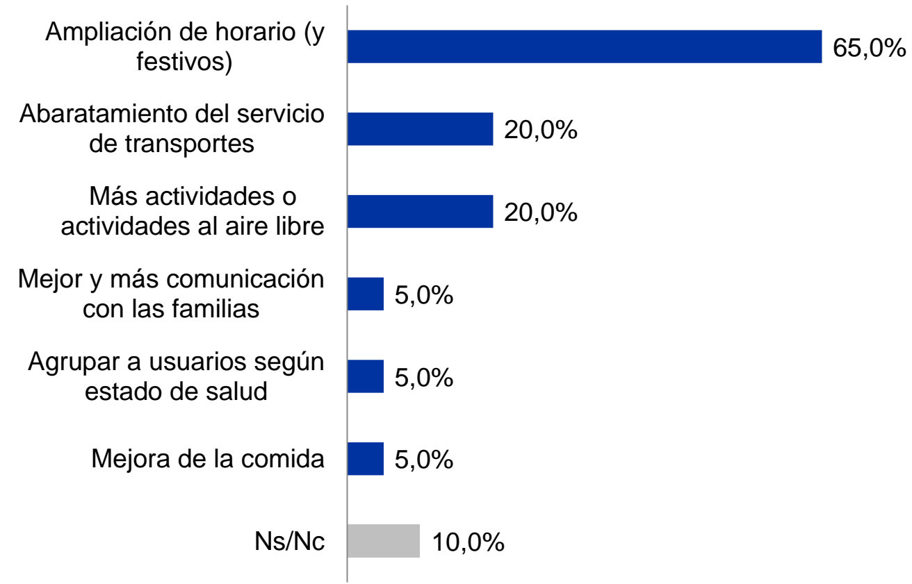
Base=20
