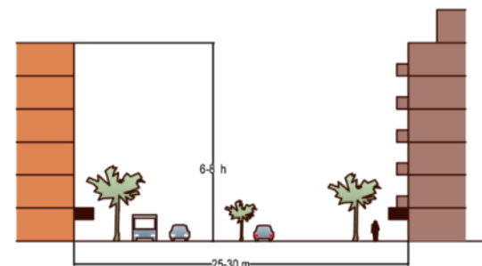
Sección característica del viario
