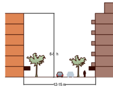
Sección característica del viario
